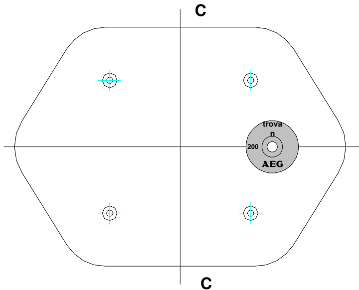
Abbildung 4.3: optimale Positionierung des Transponders über der Antenne (statisch)
