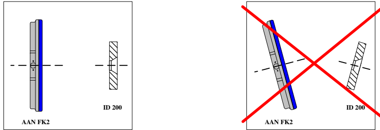
Abbildung 4.1: optimale Ausrichtung Transponder - Antenne
