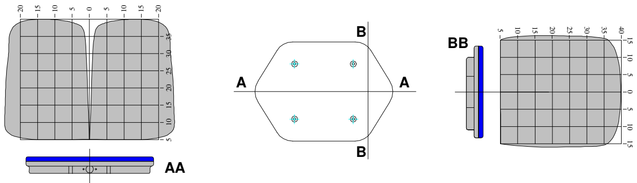
Abbildung 4.2: Lesefeld für ID200 oberhalb der Längsachse (AA) und der Querachse (BB)
